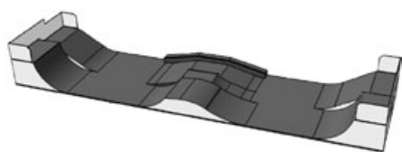
Monolitický skatepark o rozměrech 25 × 6,6 m. Výška bočních nástupních ploch max. 1,9 m.
